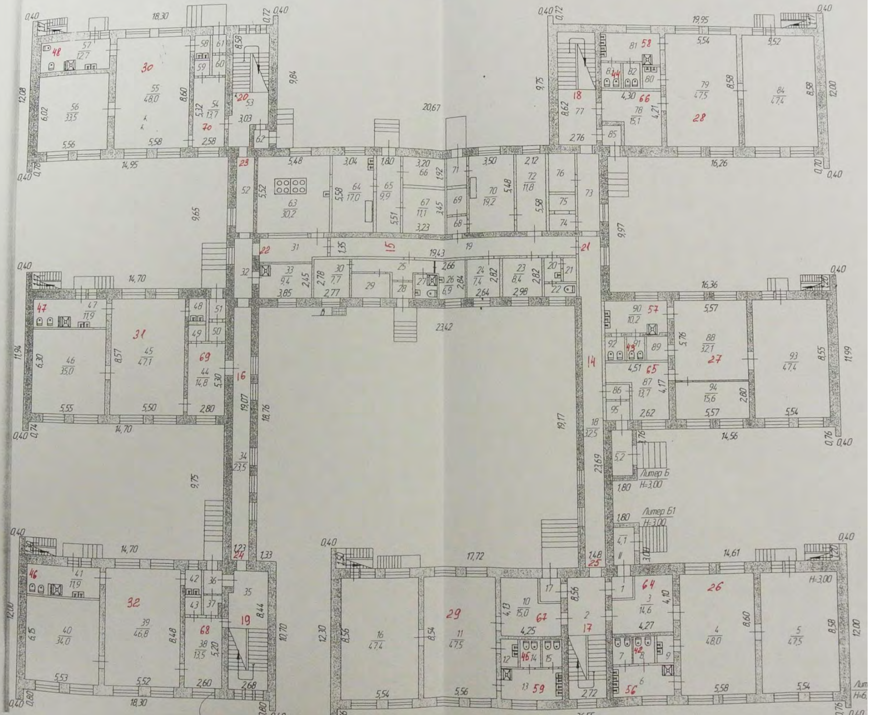
План 7 этажа
